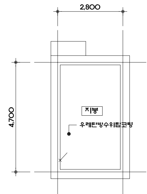
옥탑지붕 평면도 scale:1/100
